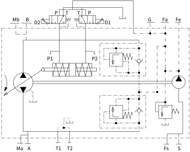
V40D23 泵原理图
